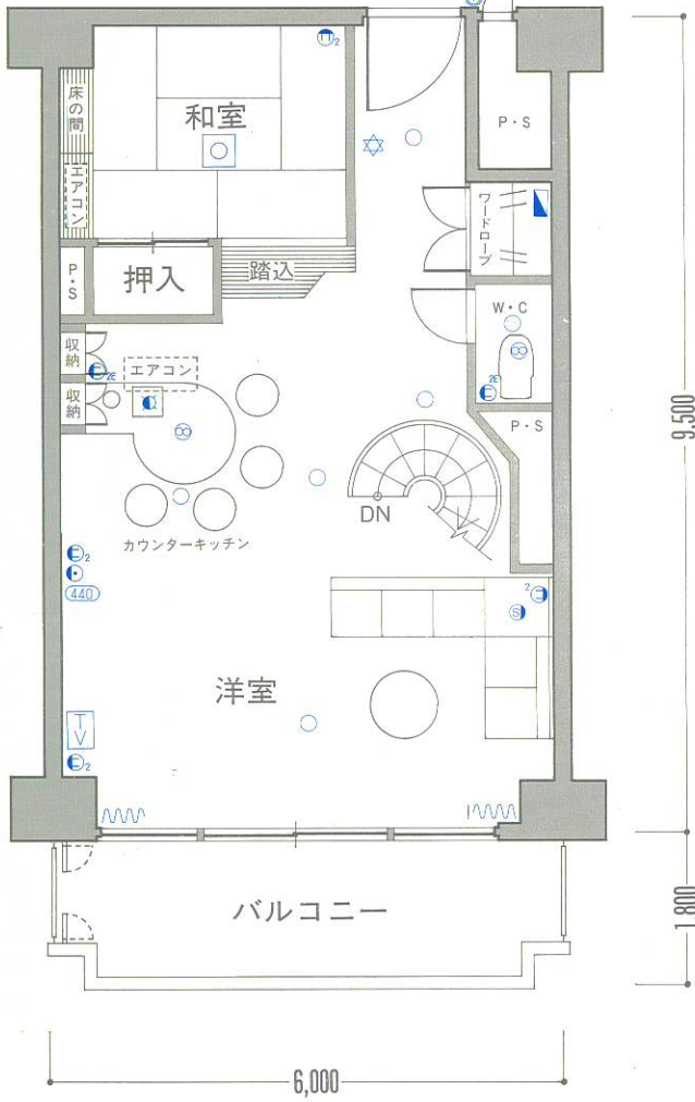
(下階)
